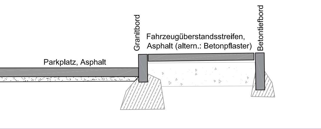
B-B'Prinzipschnitt Erweiterung Bestand
