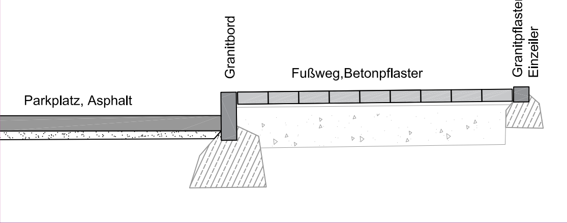
A-A'Prinzipschnitt Fußweg-Parkplatz neu
