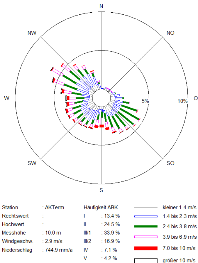
Abbildung 7: Darstellung der Häufigkeitsverteilung der Windrichtung [%] für den Windgeberstandort
