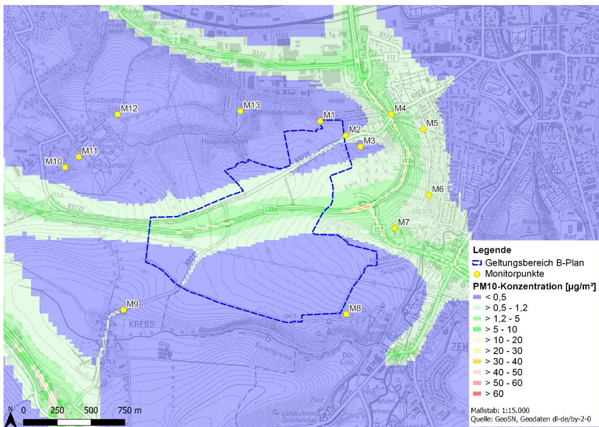
Abbildung 10: verkehrsbedingte Immissionszusatzbelastung (IZ) der \text{PM}_{10} -Konzentration im Prognose-Nullfall mit Berücksichtigung von Kaltlufteinflüssen
