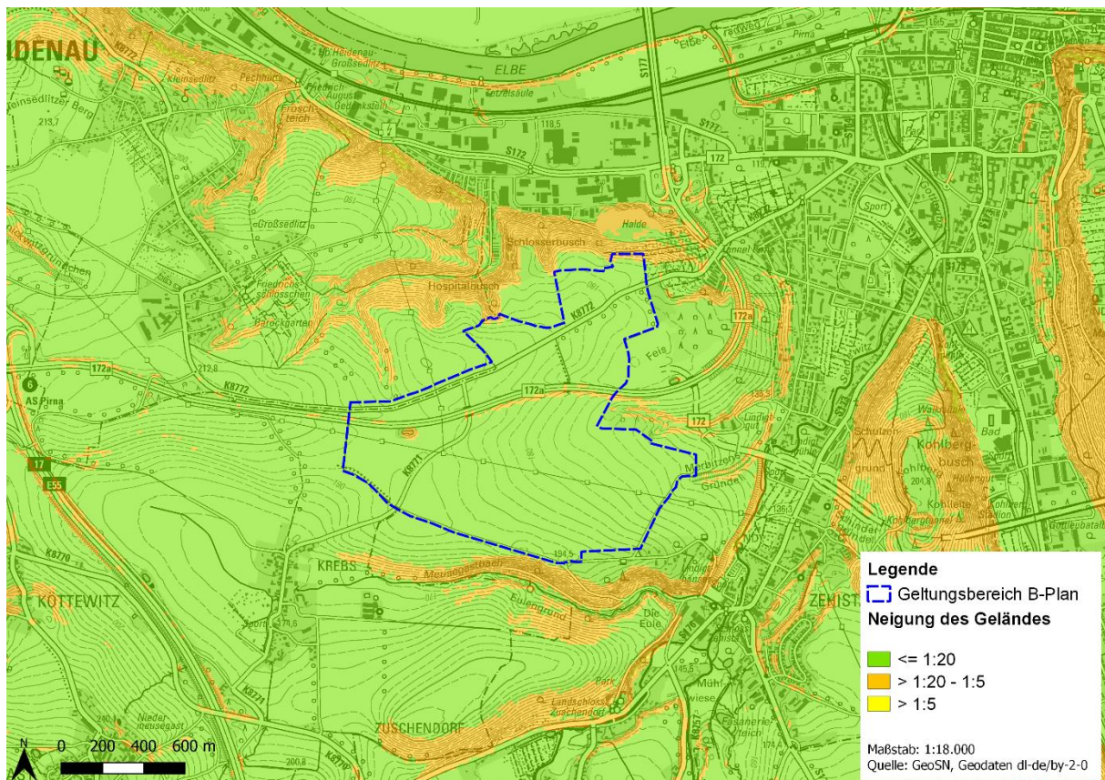
Abbildung 6: Neigung des Geländes im Untersuchungsraum
