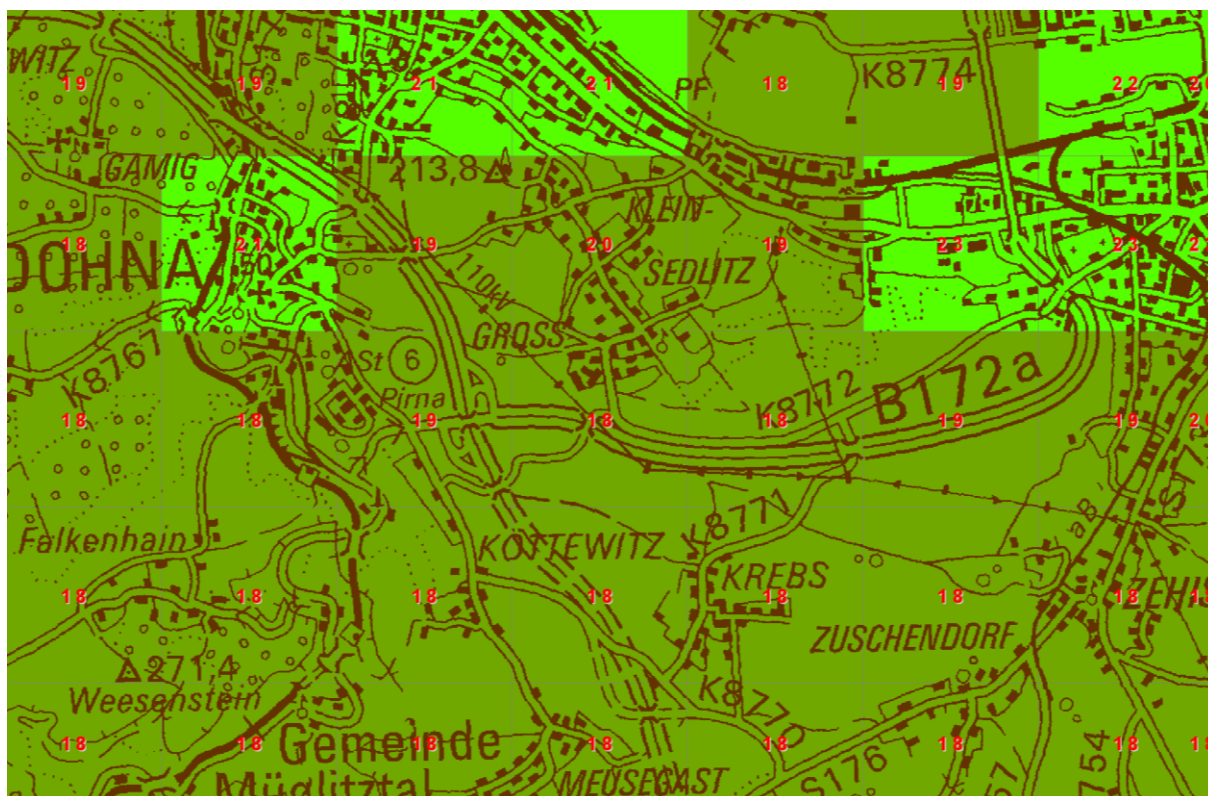
Abbildung 3.2: Hintergrundbelastung der PM 10 -Konzentration [µg/m³] im Untersuchungsraum [2]
