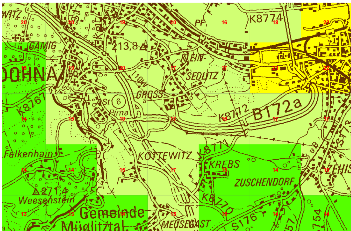
Abbildung 3.1: Hintergrundbelastung der NO 2 -Konzentration [µg/m³] im Untersuchungsraum [2]
