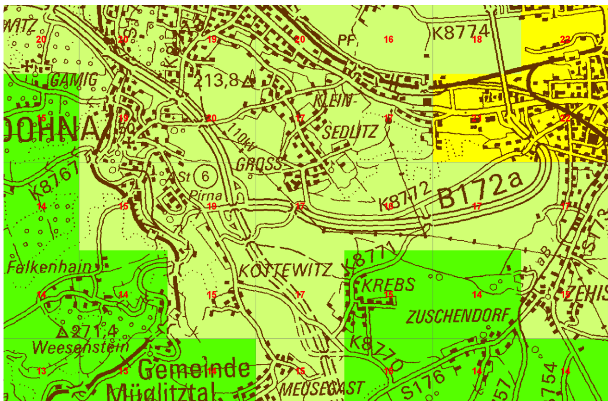
Abbildung 4: Hintergrundbelastung der NO 2 -Konzentration [ \mu\text{g}/\text{m}^3 ] im Untersuchungsraum [6]
