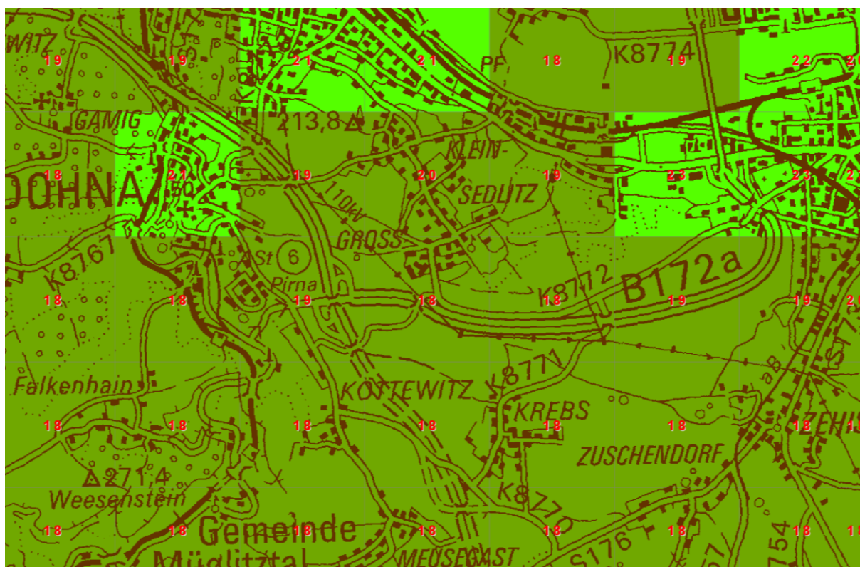
Abbildung 5: Hintergrundbelastung der PM 10 -Konzentration [ \mu\text{g}/\text{m}^3 ] im Untersuchungsraum [6]
