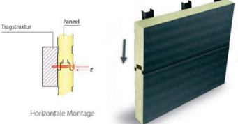
2_ Sandwich-Panel Fassade, horizontale Befestigung zwischen Stützen in Farbton RAL 5009 Auszubau Panel Breite: 1,20m
