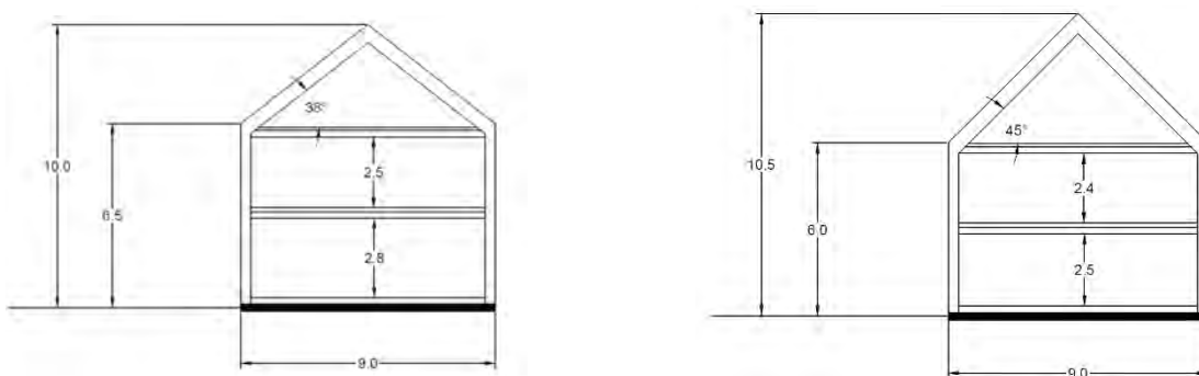
Abb. 4: Prinzipschnitte Wohngebäude
