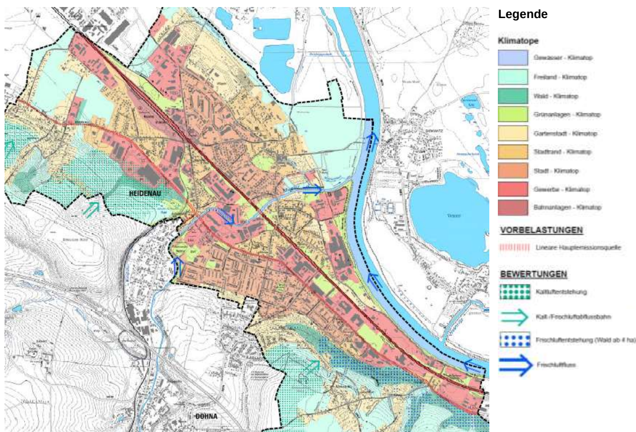
Abb. 13: Landschaftsplan Heidenau, Potentialkarte Schutzgut Klima (Entwurf), Ausschnitt
