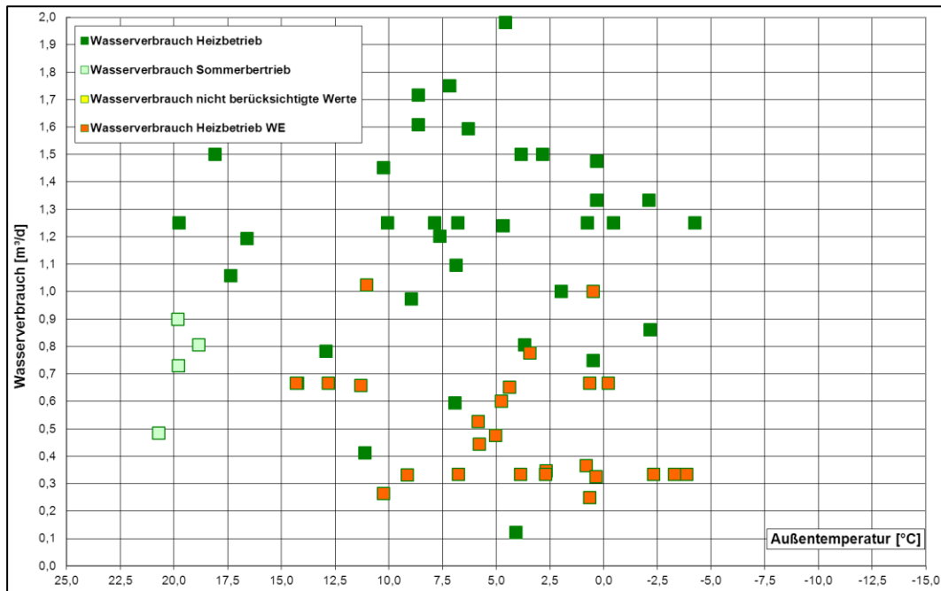
Bild 24: Heinrich-Heine-Grundschule - Wasserverbrauch in Abhängigkeit von der Außentemperatur
