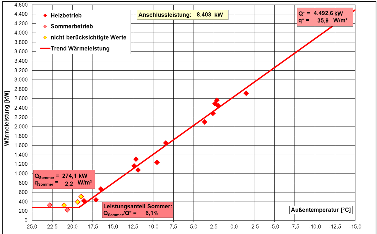
Bild 37: Wärmeleistung in Abhängigkeit von der Außentemperatur für Heizhaus Beethovenstraße
