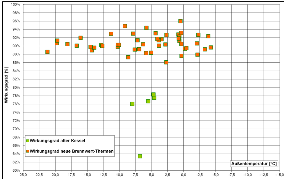
Bild 29: Kesselwirkungsgrad für den alten Kessel und die neuen Brennwert-Thermen
