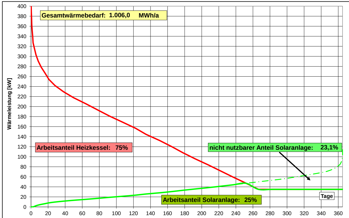
Bild 36: geordnete Jahresdauerlinie der Wärmeleistung für Solaranlage mit 25 % Arbeitsanteil
