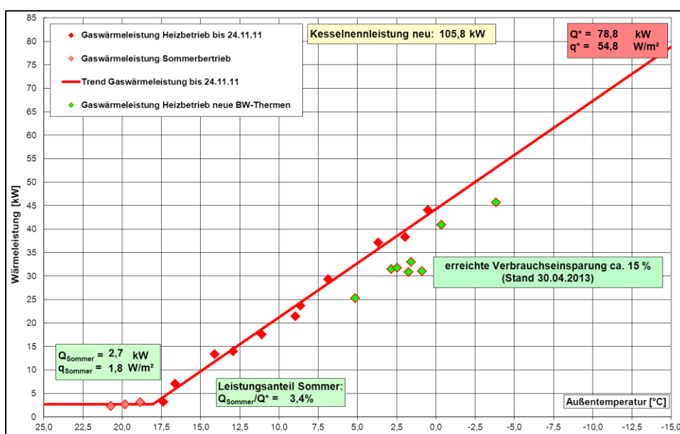
Bild 28: Verbrauchseinsparungen nach Austausch des alten Kessels durch zwei Brennwert-Thermen
