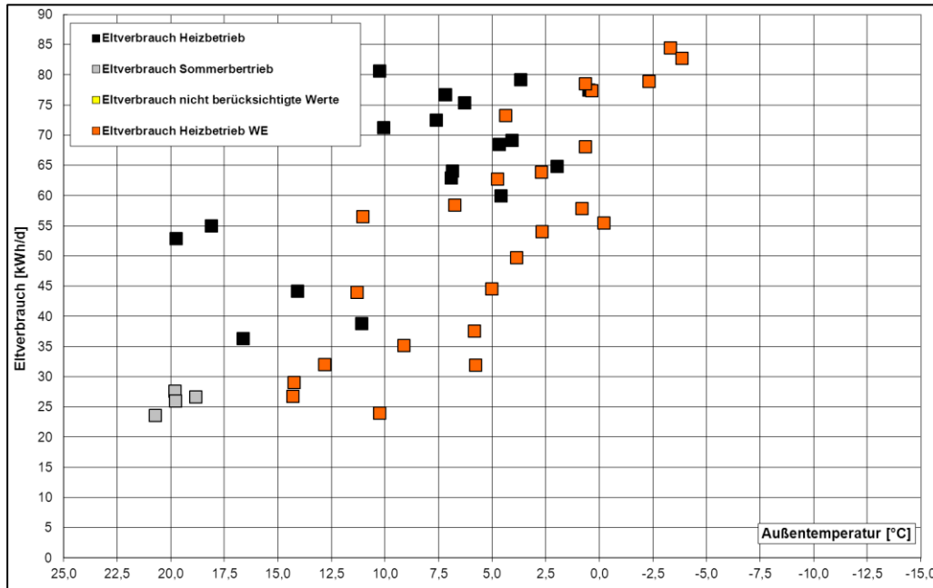
Bild 23: Heinrich-Heine-Grundschule - Elektroenergieverbrauch in Abhängigkeit von der Außentemperatur
