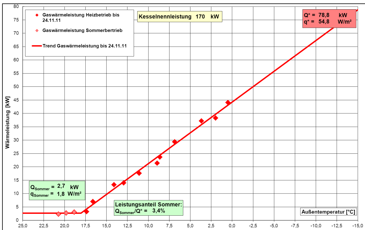
Bild 22: Heinrich-Heine-Grundschule – Brennstoff-Wärmeleistung in Abhängigkeit von der Außentemperatur
