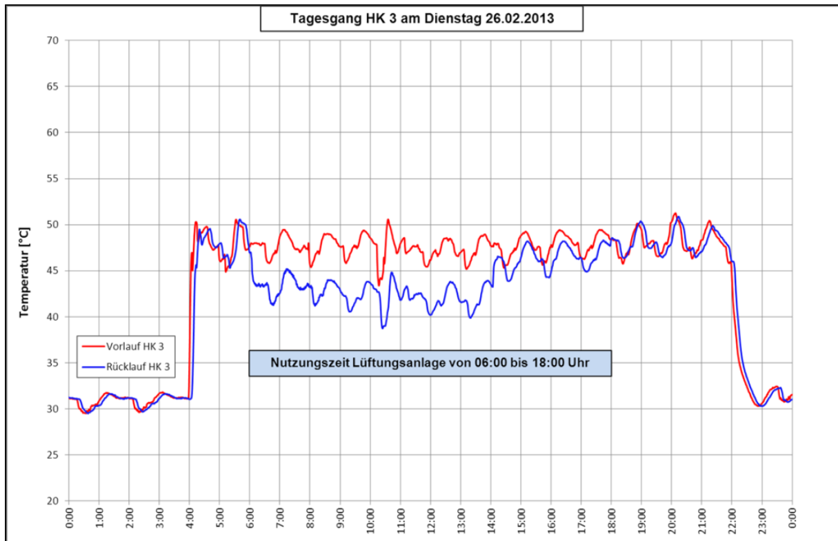
Bild 31: Lüftungskreis nach Optimierung
