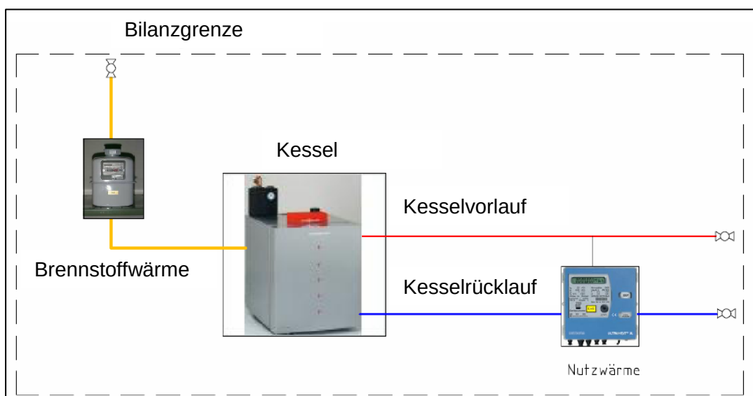
Bild 34: Brennstoffwärme und Nutzwärme
