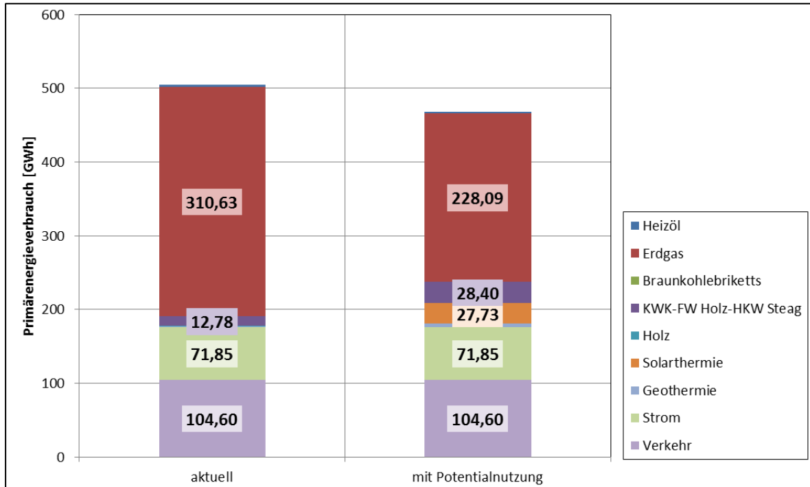
Bild 18: Primärenergieverbrauch ohne und mit Nutzung der Potenziale
