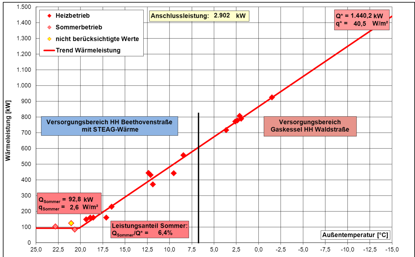
Bild 38: Wärmeleistung in Abhängigkeit von der Außentemperatur für Heizhaus Waldstraße
