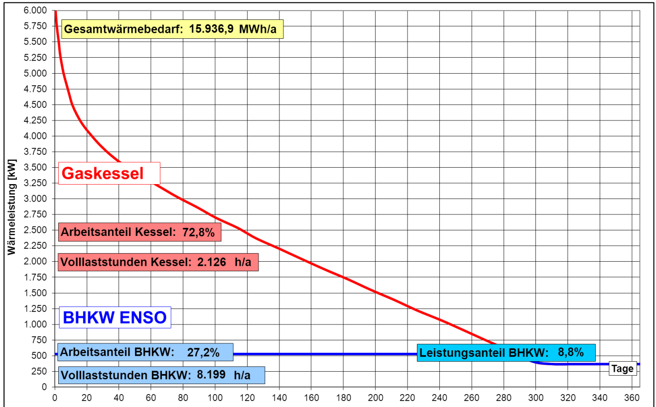
Bild 41: Jahresdauerlinie für den Absatz in beide Netz WUS mit Einordnung des BHKW
