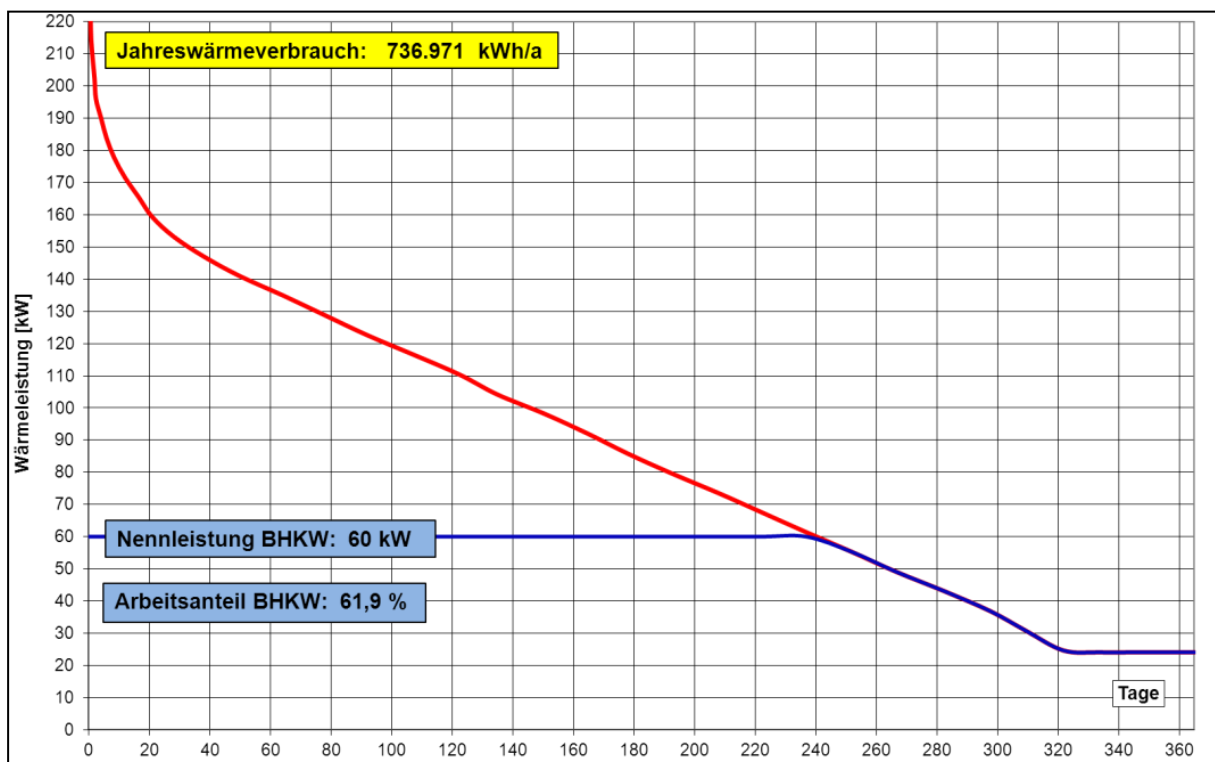
Bild 35: geordnete Jahresdauerlinie der Wärmeleistung für BHKW und Spitzenlastkessel
