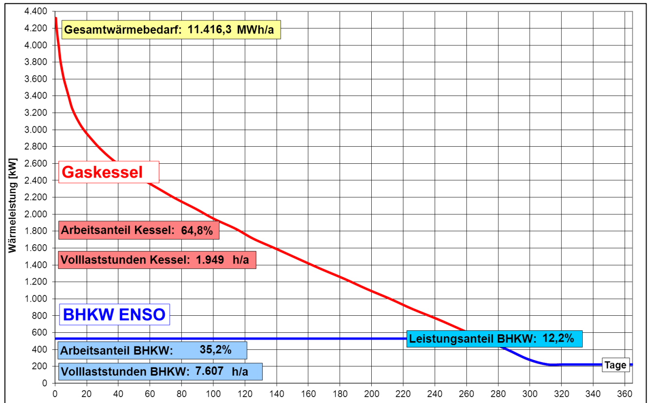
Bild 40: Jahresdauerlinie für den Absatz im Netz des Heizhaus Beethovenstraße mit Einordnung des BHKW
