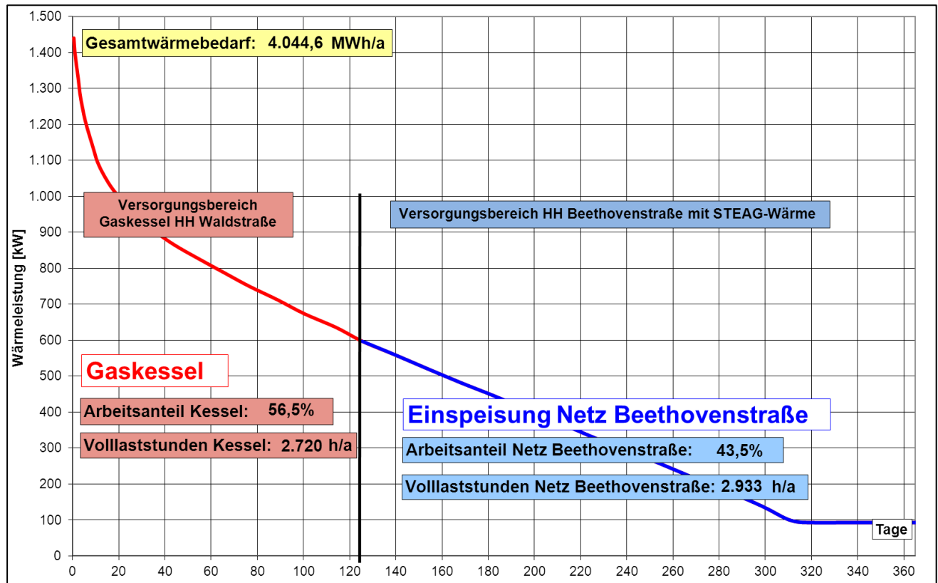
Bild 39: Jahresdauerlinie für die Abnehmer des Heizhauses Waldstraße mit Einordnung der „STEAG“-Wärme
