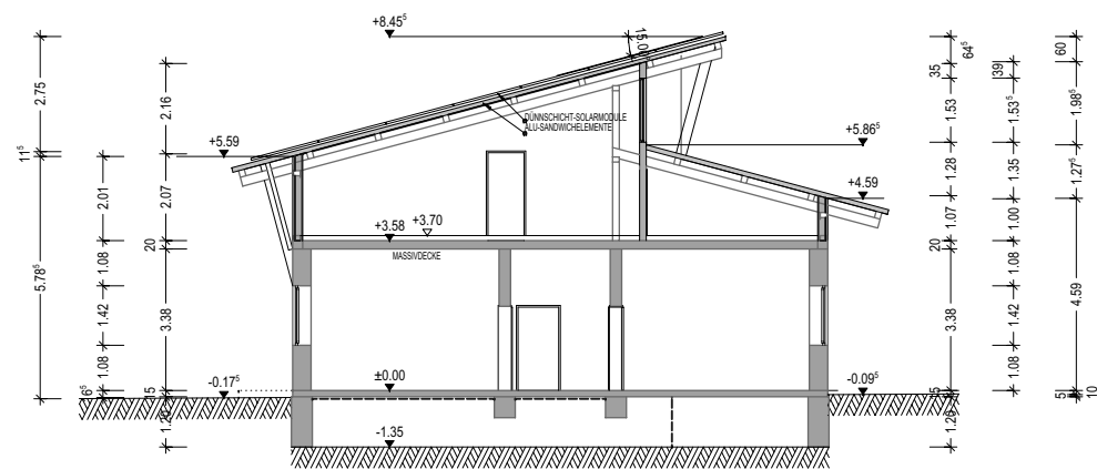
SNITT A - HAUPTGEBÄUDE
